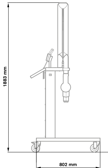
Vue latérale
