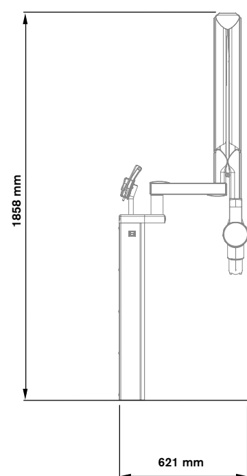
Vue latérale
