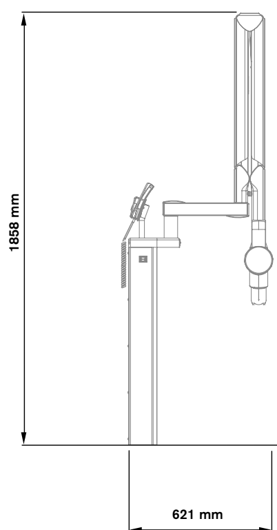
Vue latérale
