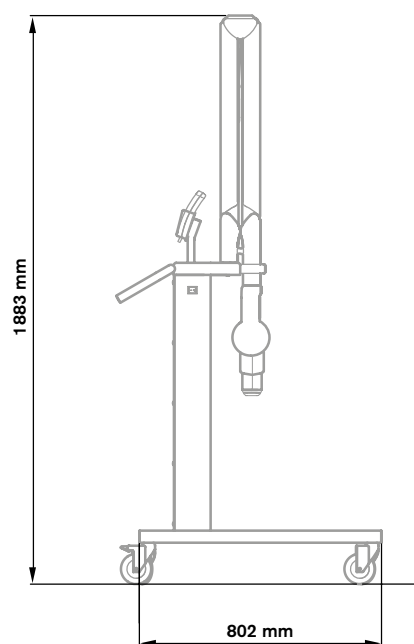
Vue latérale
