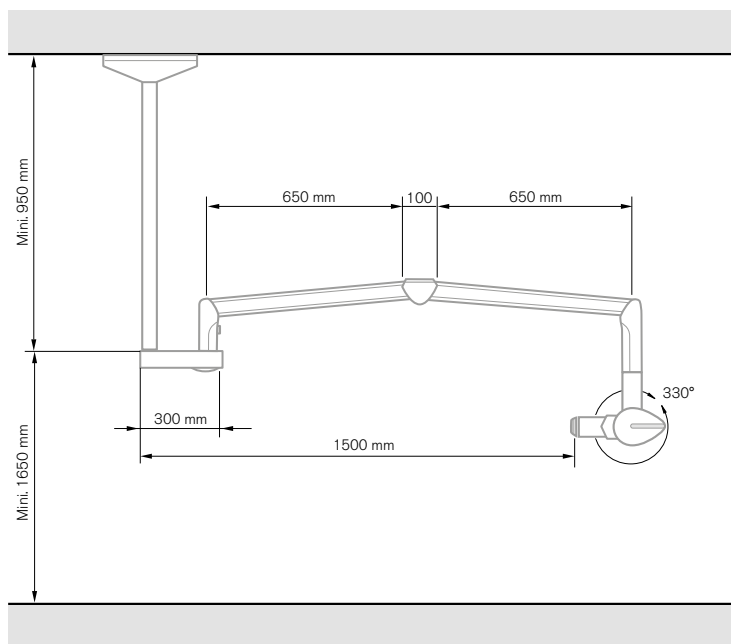
Appareil monté au plafond (bras ouvert) Vue latérale
