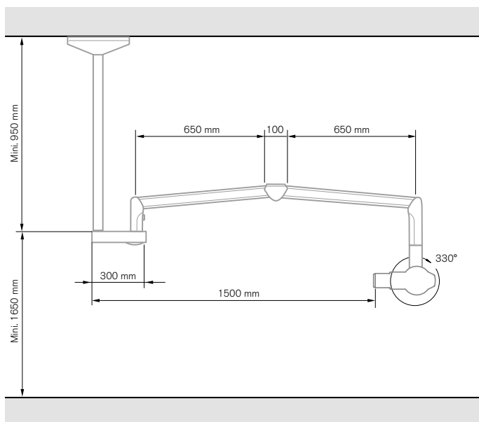
Appareil monté au plafond (bras ouvert) Vue latérale
